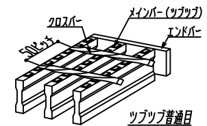
嵩上げ材詳細図
