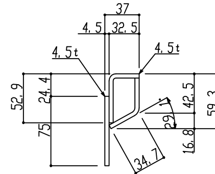
嵩上げ材詳細図
